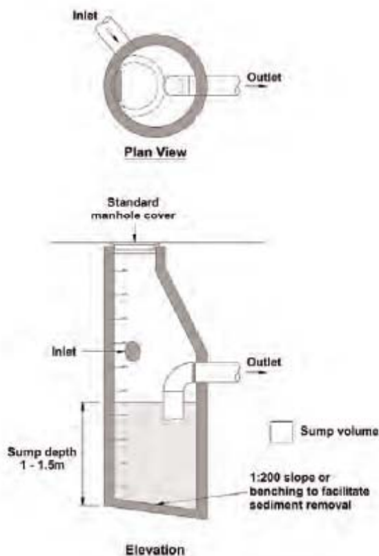
Figura 25.7- Poço de visita que é usado como pré-tratamento off line Fonte: CIRIA, 2007
