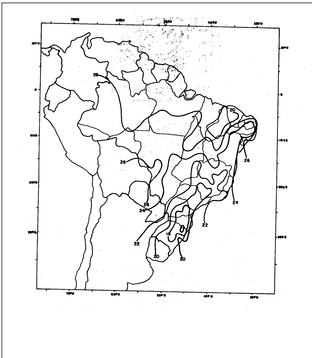
Figura 13.2- Temperatura médias anuais em graus centígrados do Brasil (1931 a 1960) Fonte: Inemet
