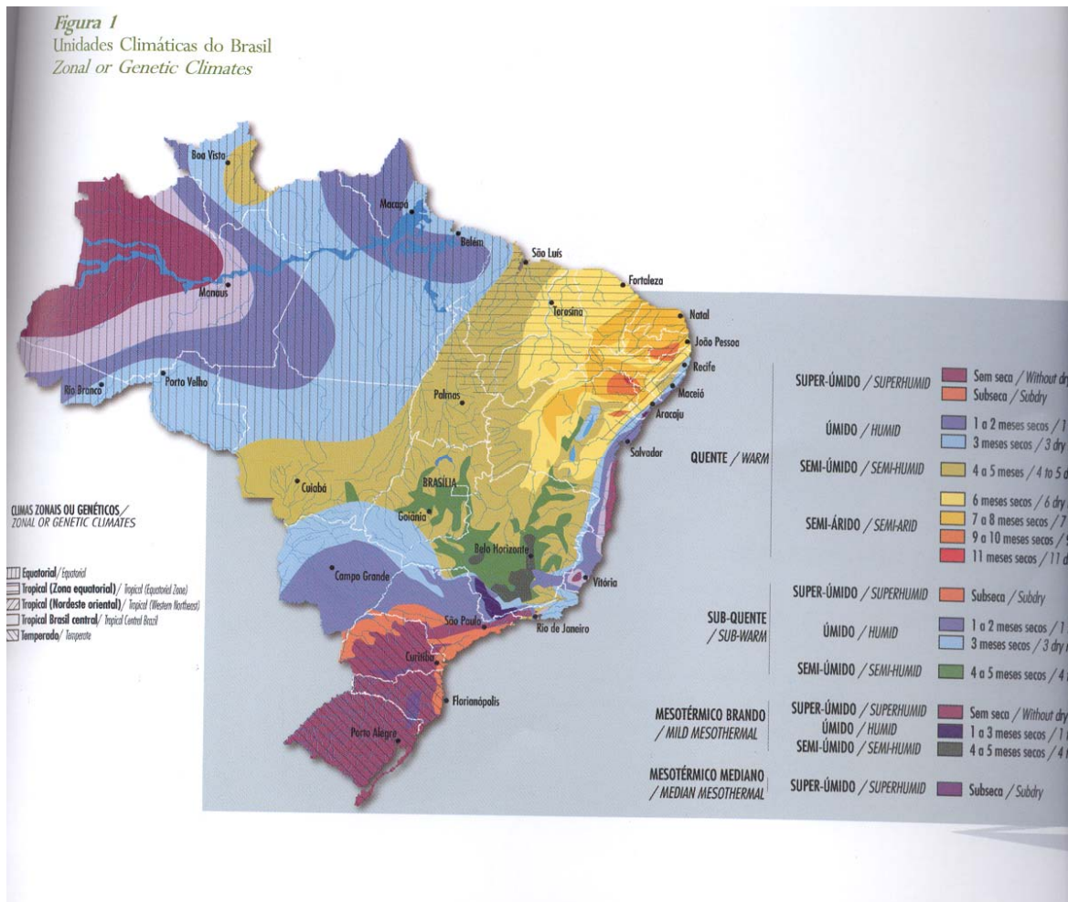
Figura 13.3- Climas do Brasil
