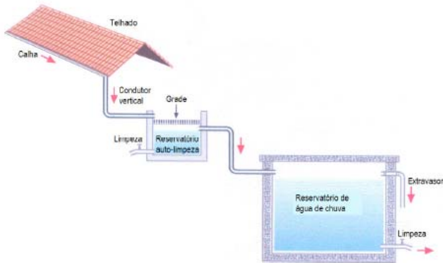
Figura 4- Esquema de funcionamento do reservatório de autolimpeza
