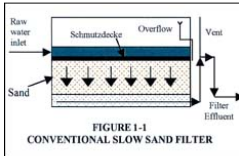
Figura 5- Esquema de um filtro lento de areia lento descendente com entrada e saída por cima em nível superior a camada de areia.
