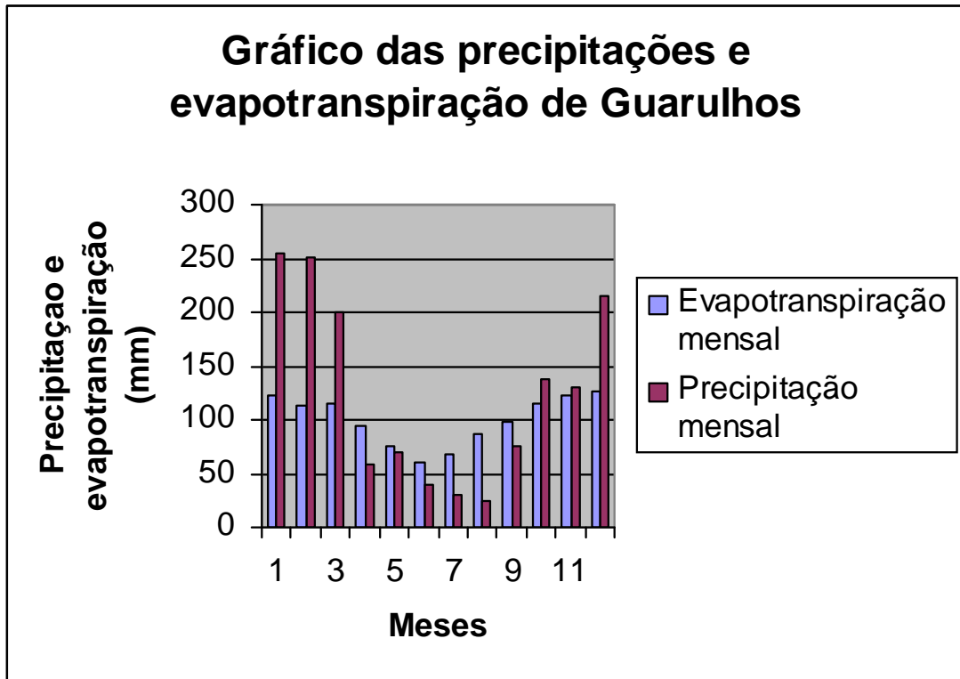
Figura 11.1- Gráfico das precipitações e evapotranspiração de referência média mensal com dados fornecidos pela UNG e aplicação do Método de Penman-Monteith, 1998 FAO.
